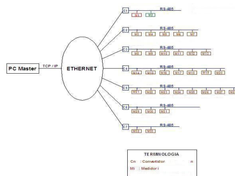
Red de medición para monitoreo centralizado de empalmes y tableros
